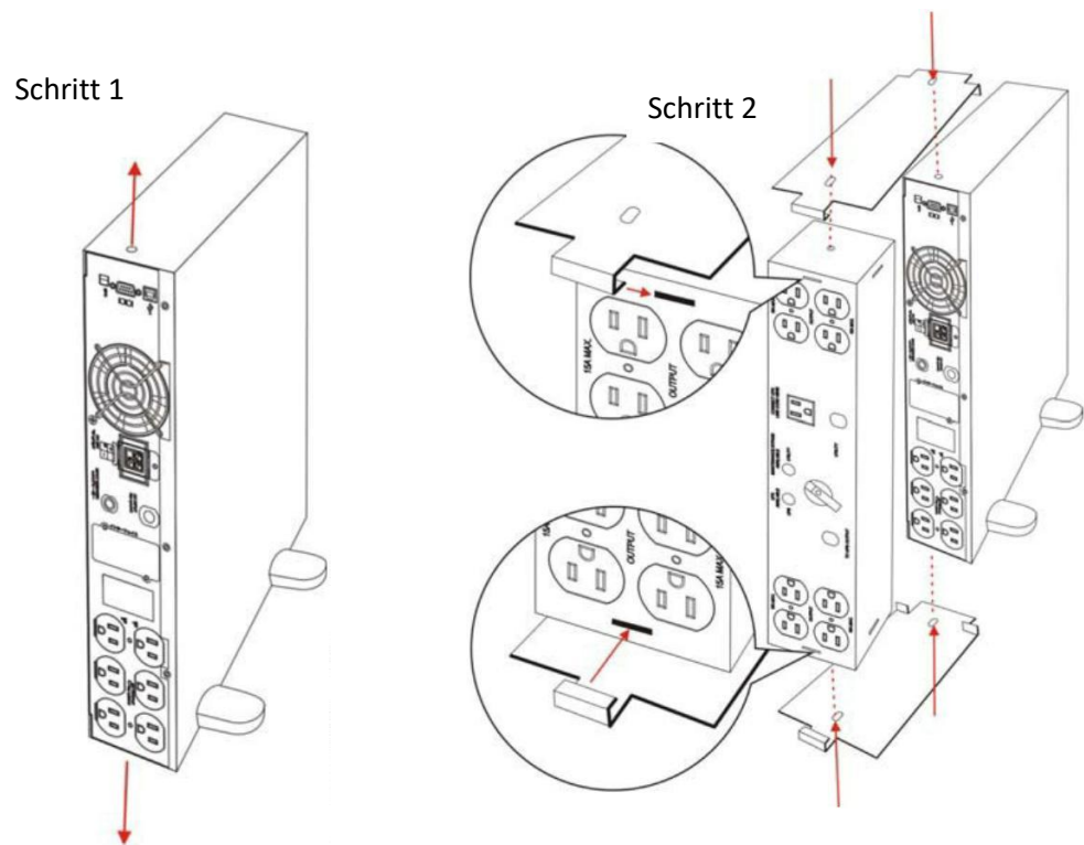
Abbildung 8: Installationsvariante (1)
