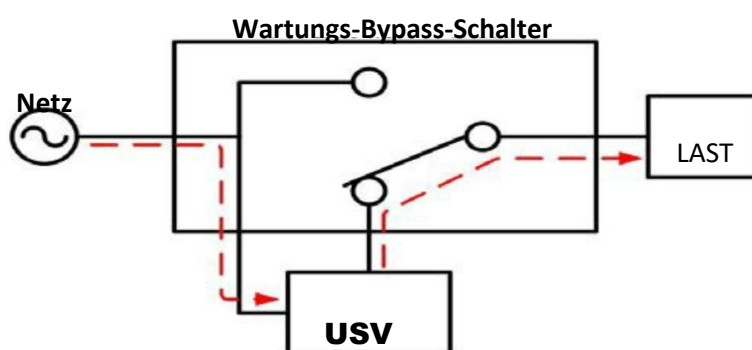
Abbildung 1: USV-Betriebsart
