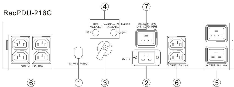
Abbildung 3: MBE Frontplatte
