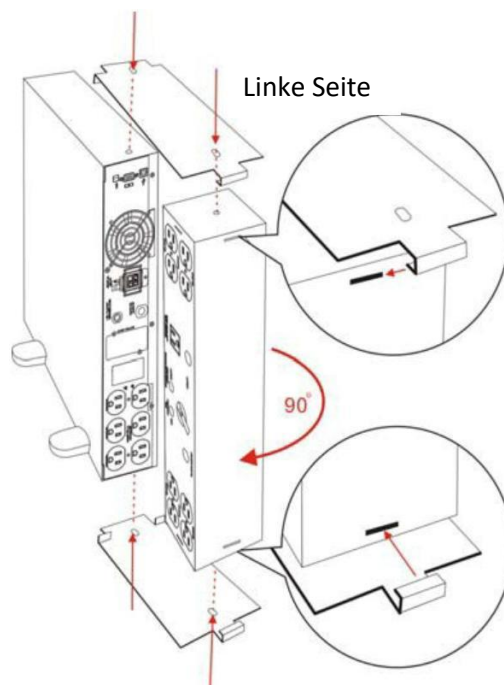
Abbildung 10: Installationsvariante (3)
