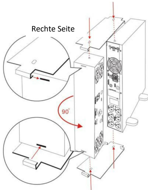
Abbildung 9: Installationsvariante (2)
