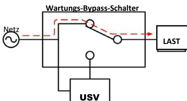
Abbildung 2: NETZ-Betriebsart
