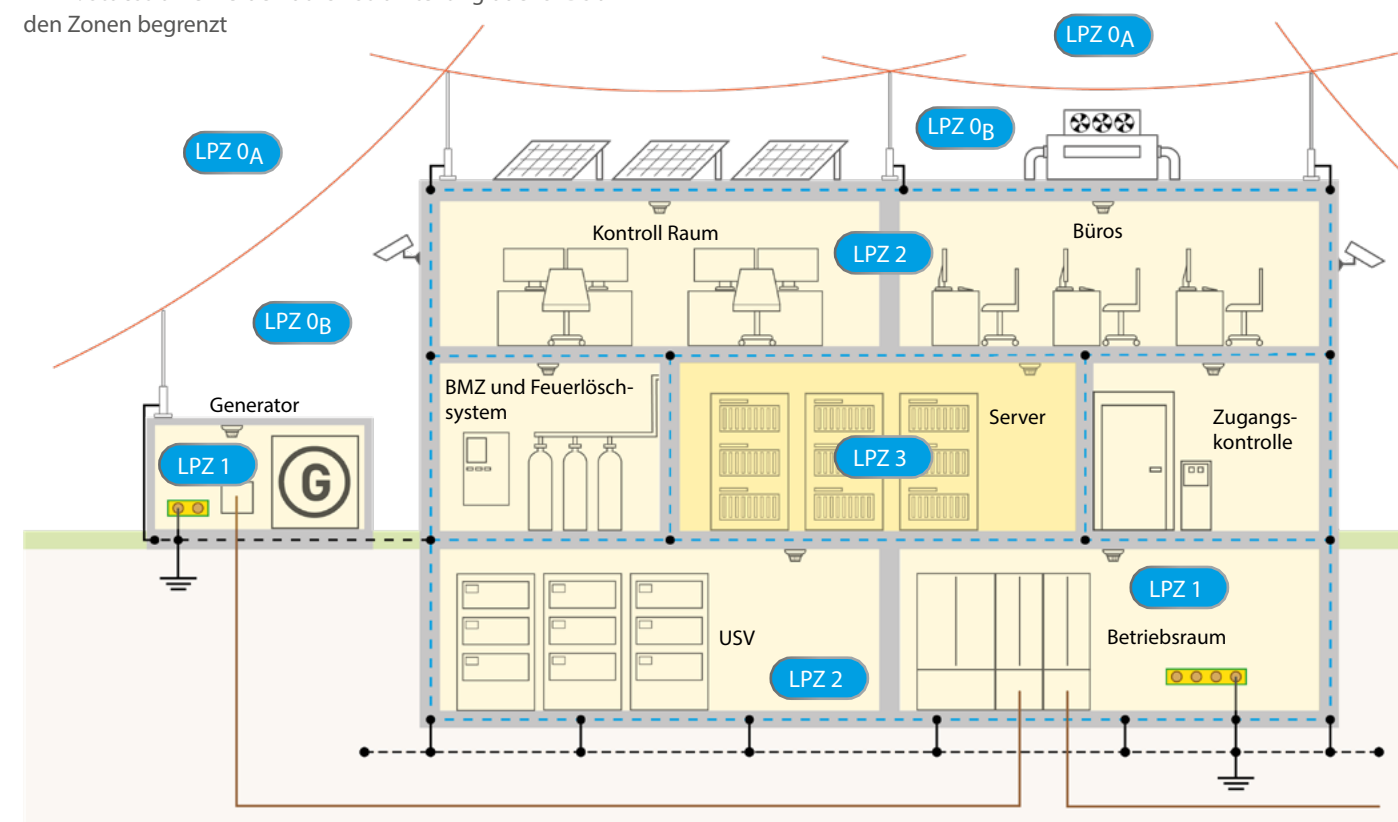
Abbildung 2: Blitzschutzzonen-Konzept
